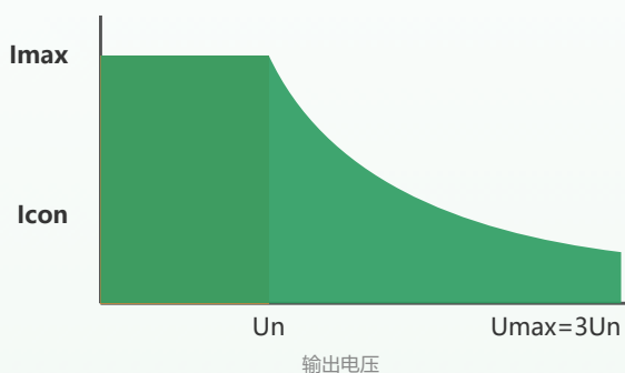
电网模拟器功率曲线图
