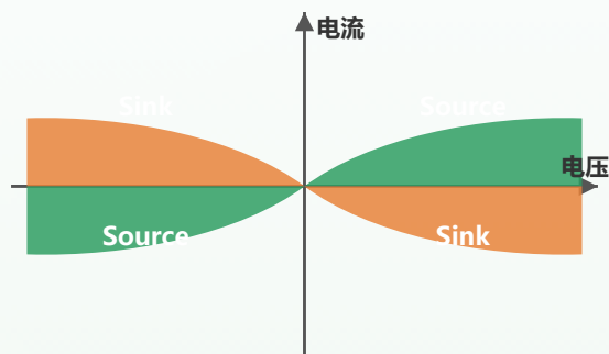
电网模拟器运行象限图
