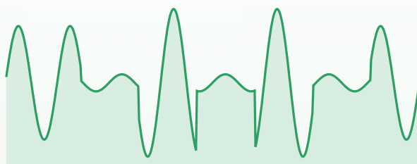
连续低-高电压穿越测试实验波形
