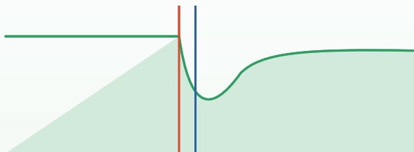
电压响应时间实验波形
